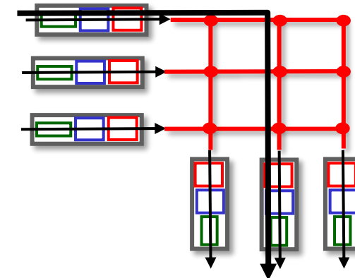
Crossbar 3x3
